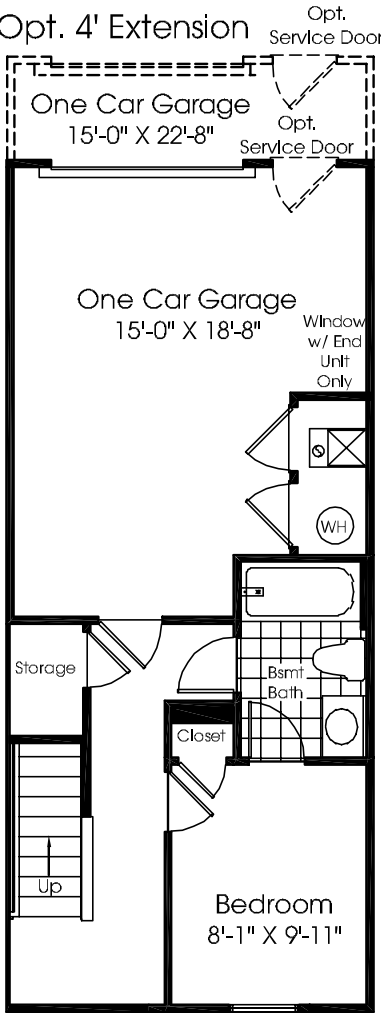
Opt. Bedroom
